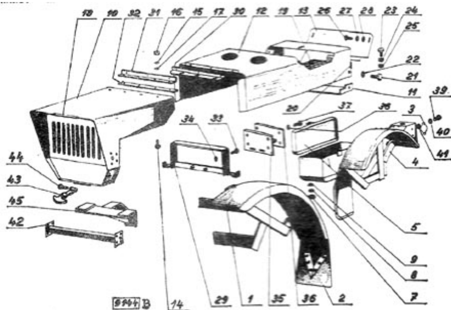
9248. Ручной тормоз.
